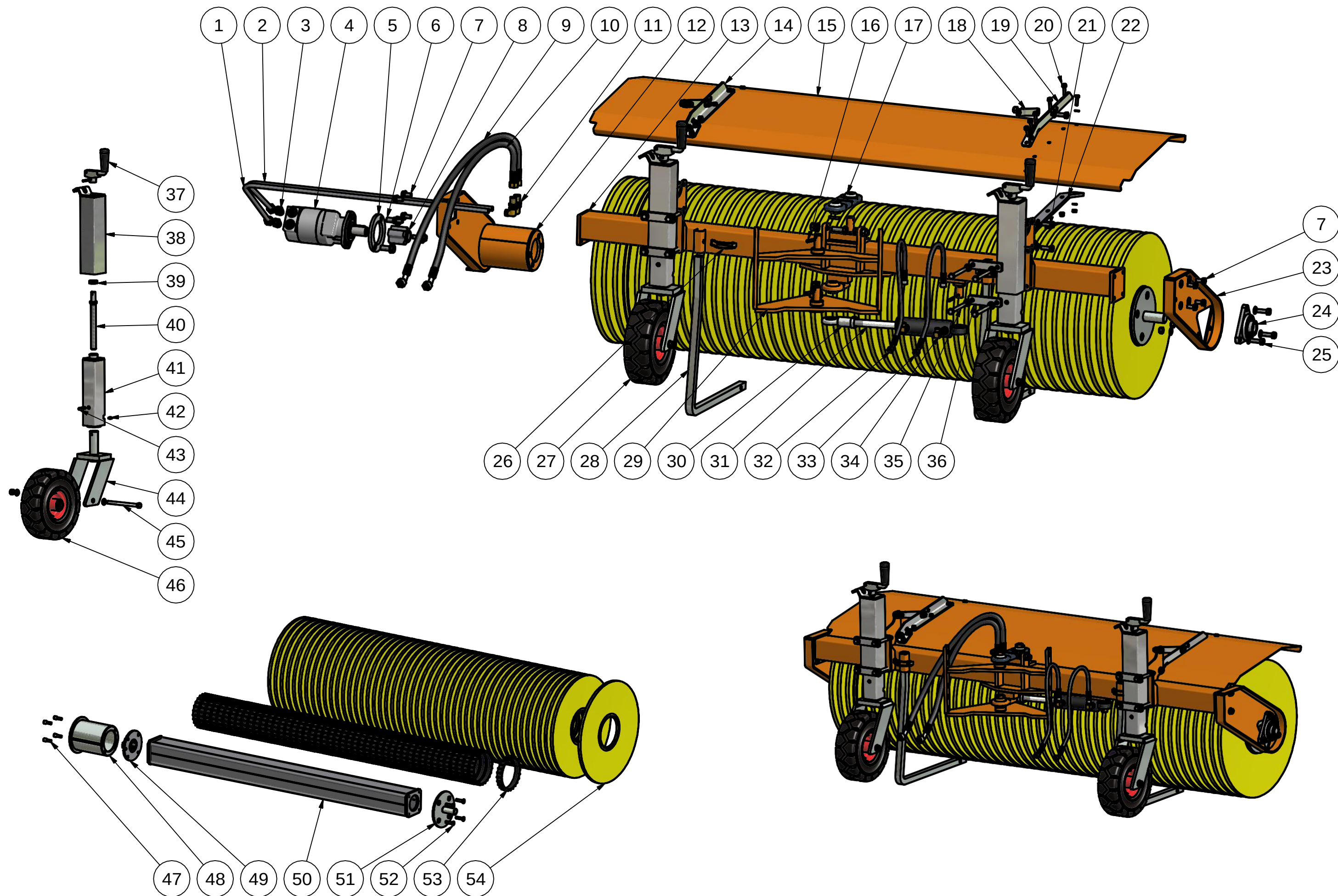
Fejemaskine HF-PL
